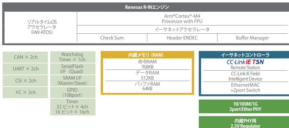
R-IN32M4-CL3 ブロック図
