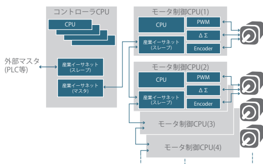
従来のシステム
