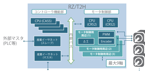
RZ/T2Hを使用したシステム
