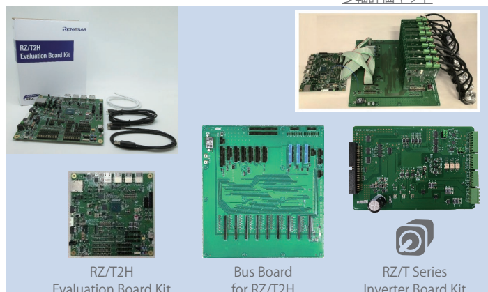
多軸評価キット
